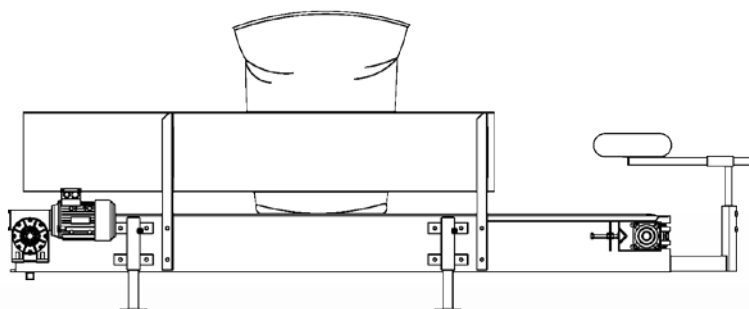
Seal / naai transportband
