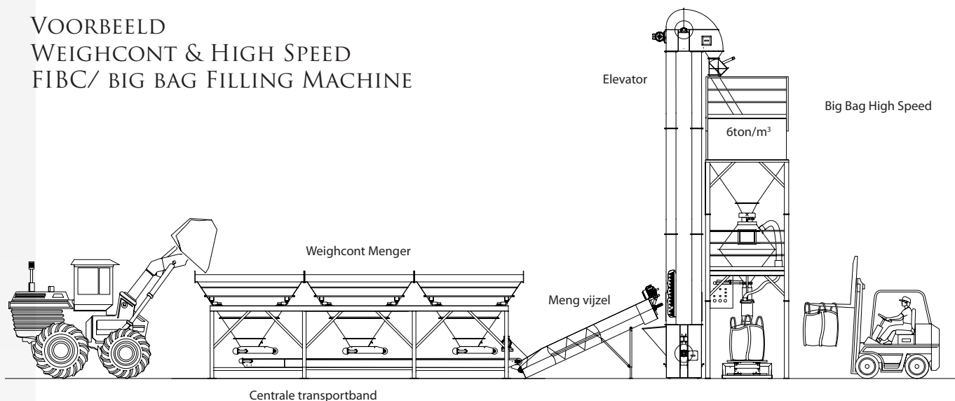
Centrale transportband
