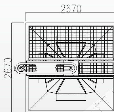
DRAUFSCICHT
